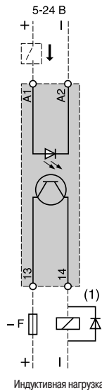
Индуктивная нагрузка
