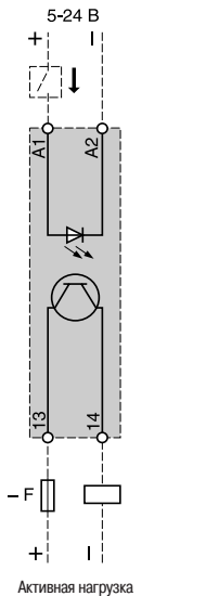
Активная нагрузка
