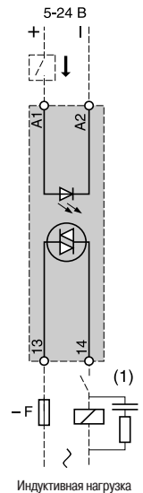
Индуктивная нагрузка
